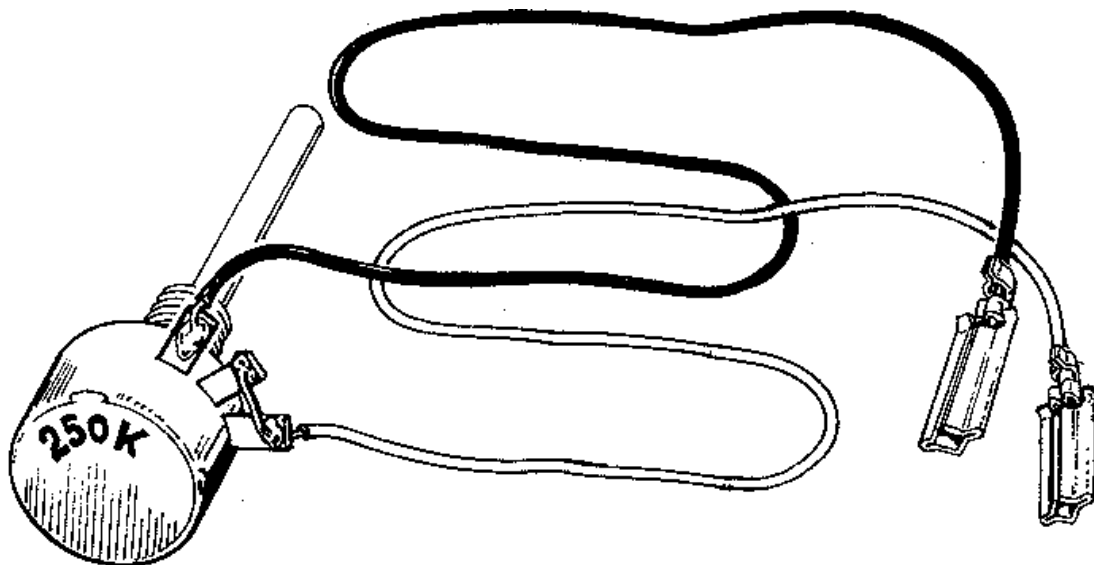
Afb. 4.5.4 De potentiometer met soldeerklemmen.
