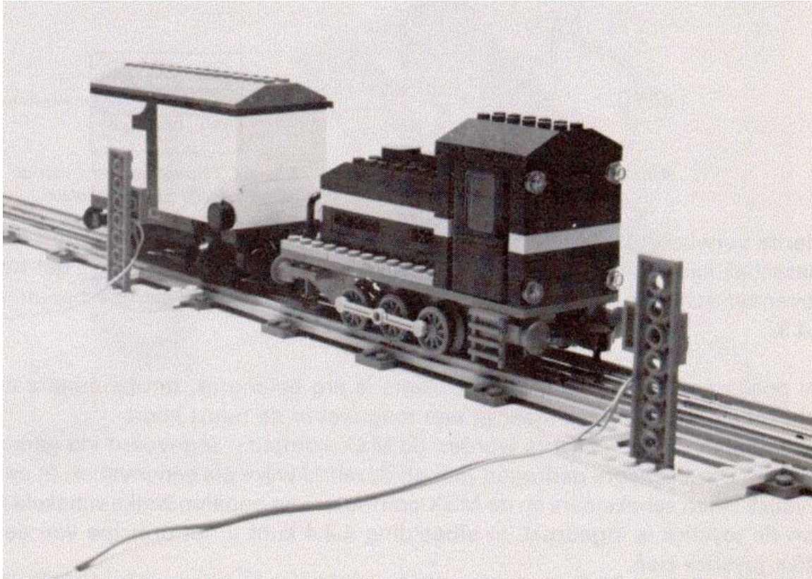
Afb. 4.4.1. De locatie van de positie sensors langs de baan. Let ook op het ronde magneetje dat op het wagentjes is gemonteerd.
