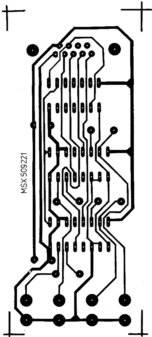
Afb. 4.5.2 De print-layout
